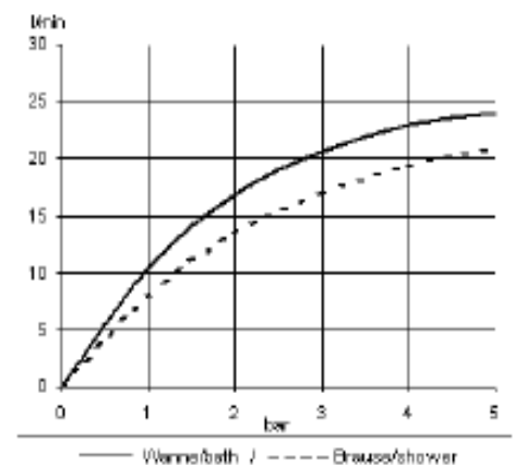
Durchflussdiagramm
