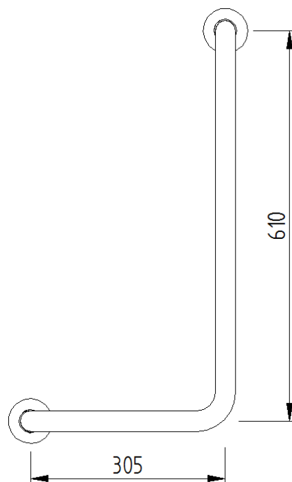
Technische Zeichnung (Ausführung Rechts)
