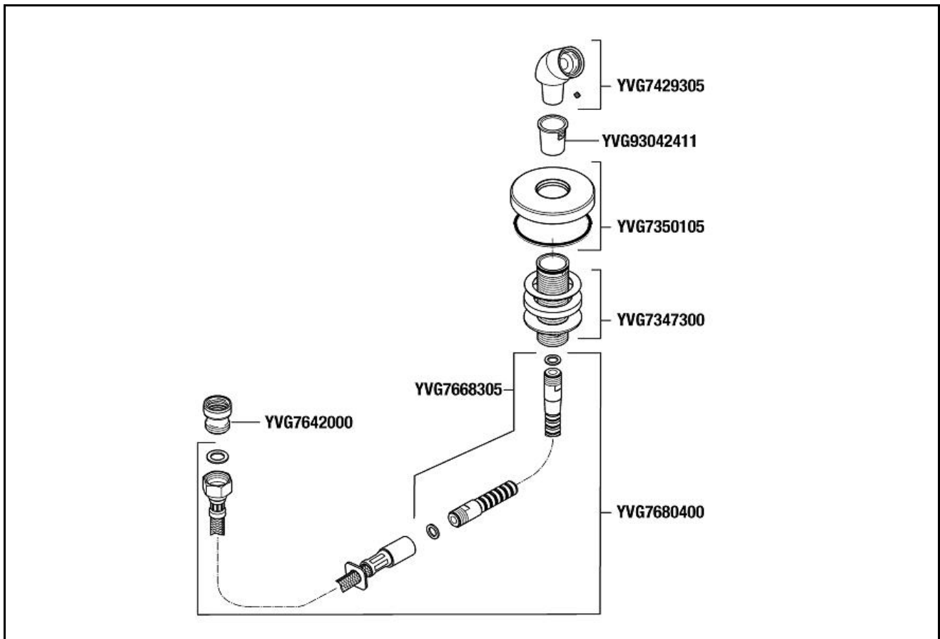
DEWRBH Wannenrandbrausehalter derby ohne Handbrause Rosette rund verchromt VIGOUR tub rim shower holder derby without Handshower Escutcheon round chr. VIGOUR
