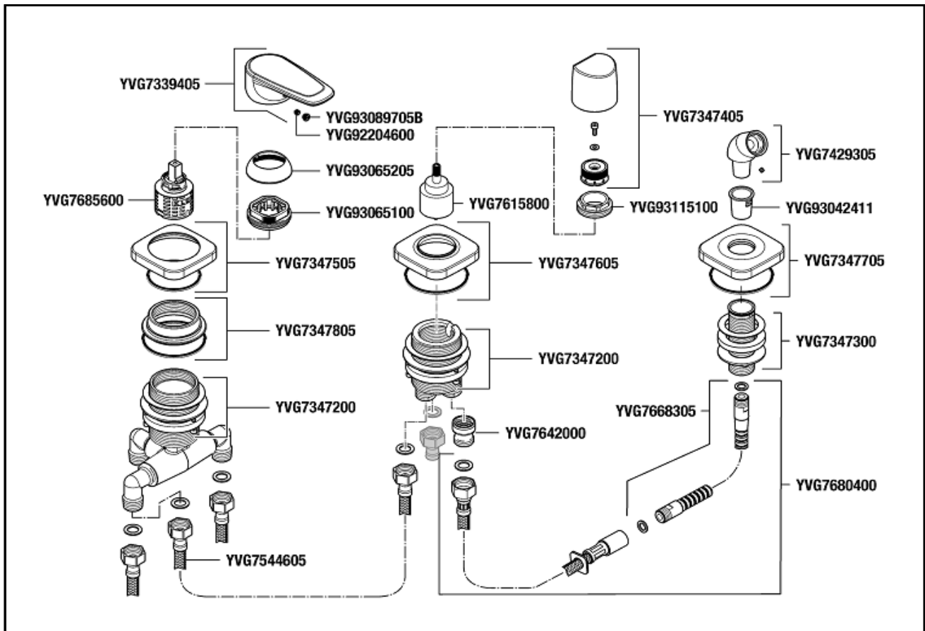
DESWF3E Dreiloch-Badebatterie derby style für entferntl. Einlauf ohne Handbrause VIG. 3-hole basin mixer derby style distant inlet without Handshower VIGOUR
